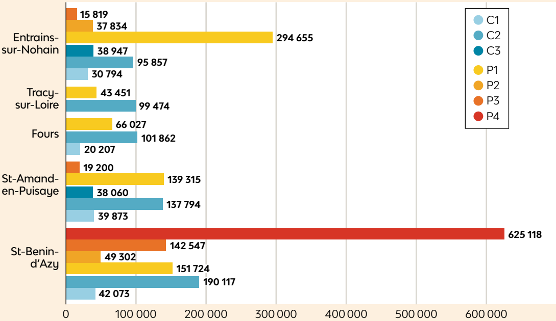
› Puissance consommée par tarif (en kW)
