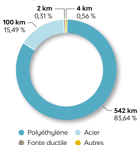
› Répartition en km des canalisations par matière, en 2025
