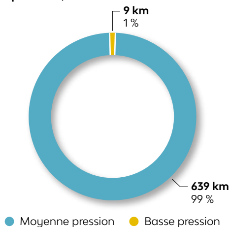
› Répartition en km des canalisations par pression, en 2025
